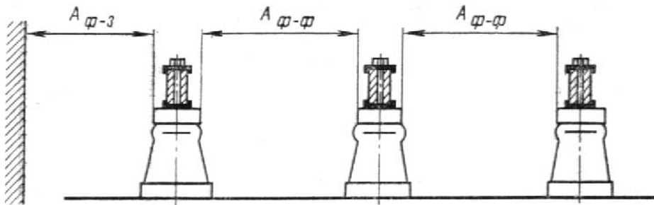
Рис. 4.2.12. Наименьшие расстояния в свету между неизолированными токоведущими частями разных фаз в ЗРУ и между ними и затолкнутыми частями (по табл. 4.2.5)
