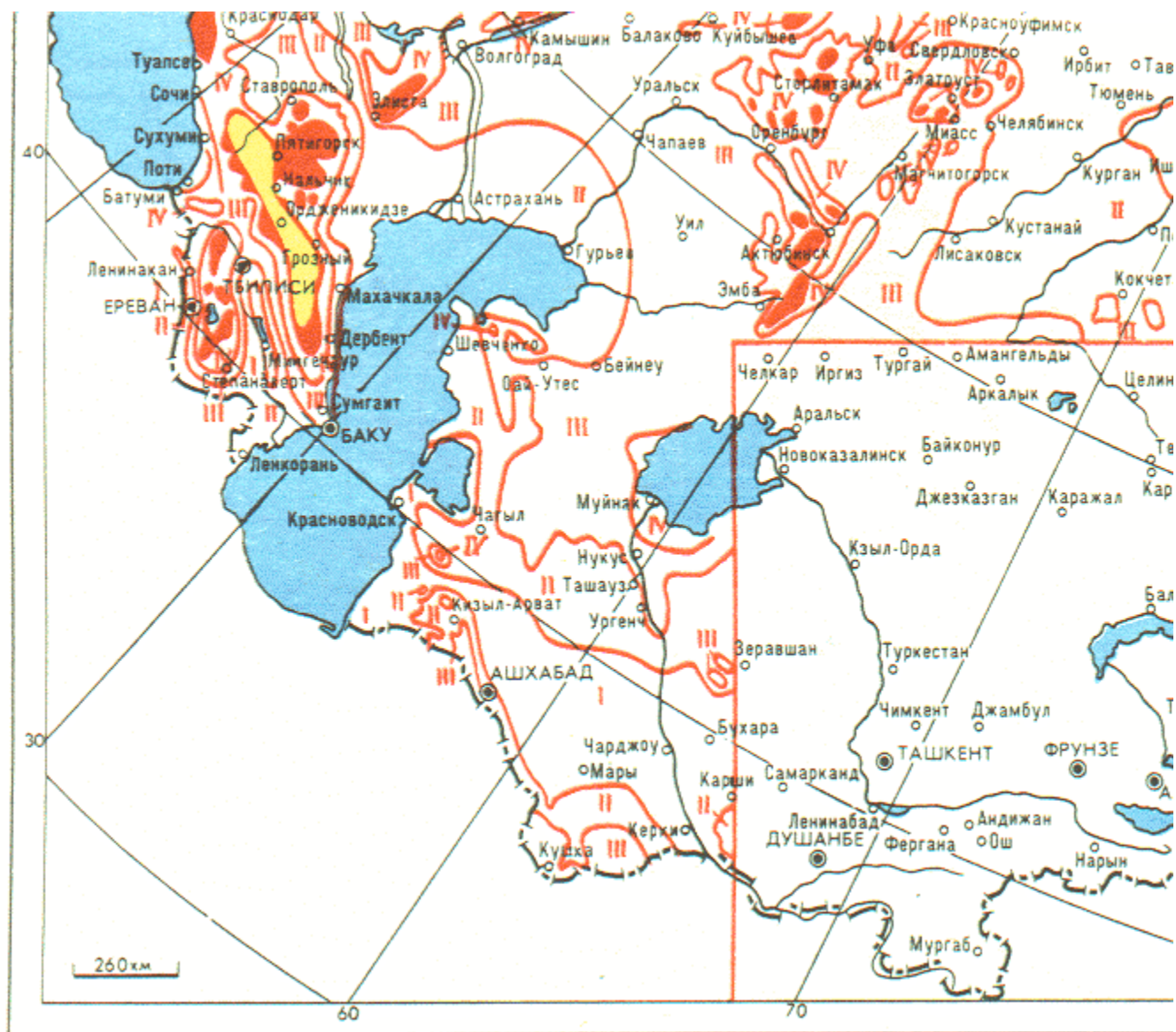
Рис. 2.5.6. Карта районирования территории СССР по толщине стенки гололеда.
