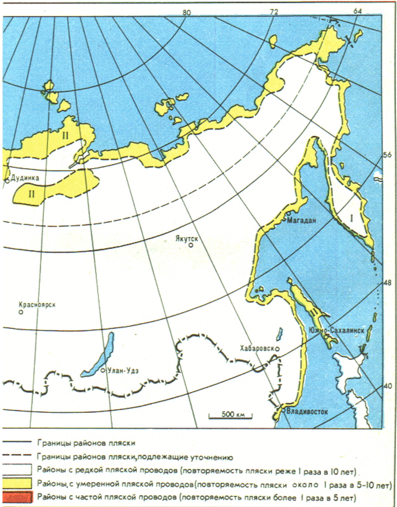
Рис. 2.5.12. Карта районирования территории СССР по пяске проводов. Лист 2
