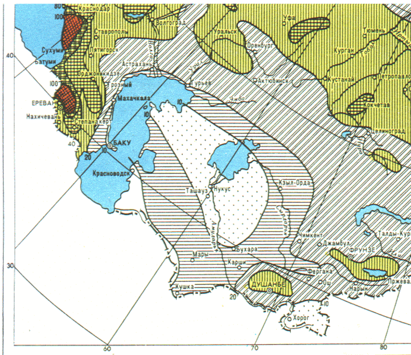
Рис. 2.5.14. Карта среднегодовой продолжительности гроз. Лист 2
