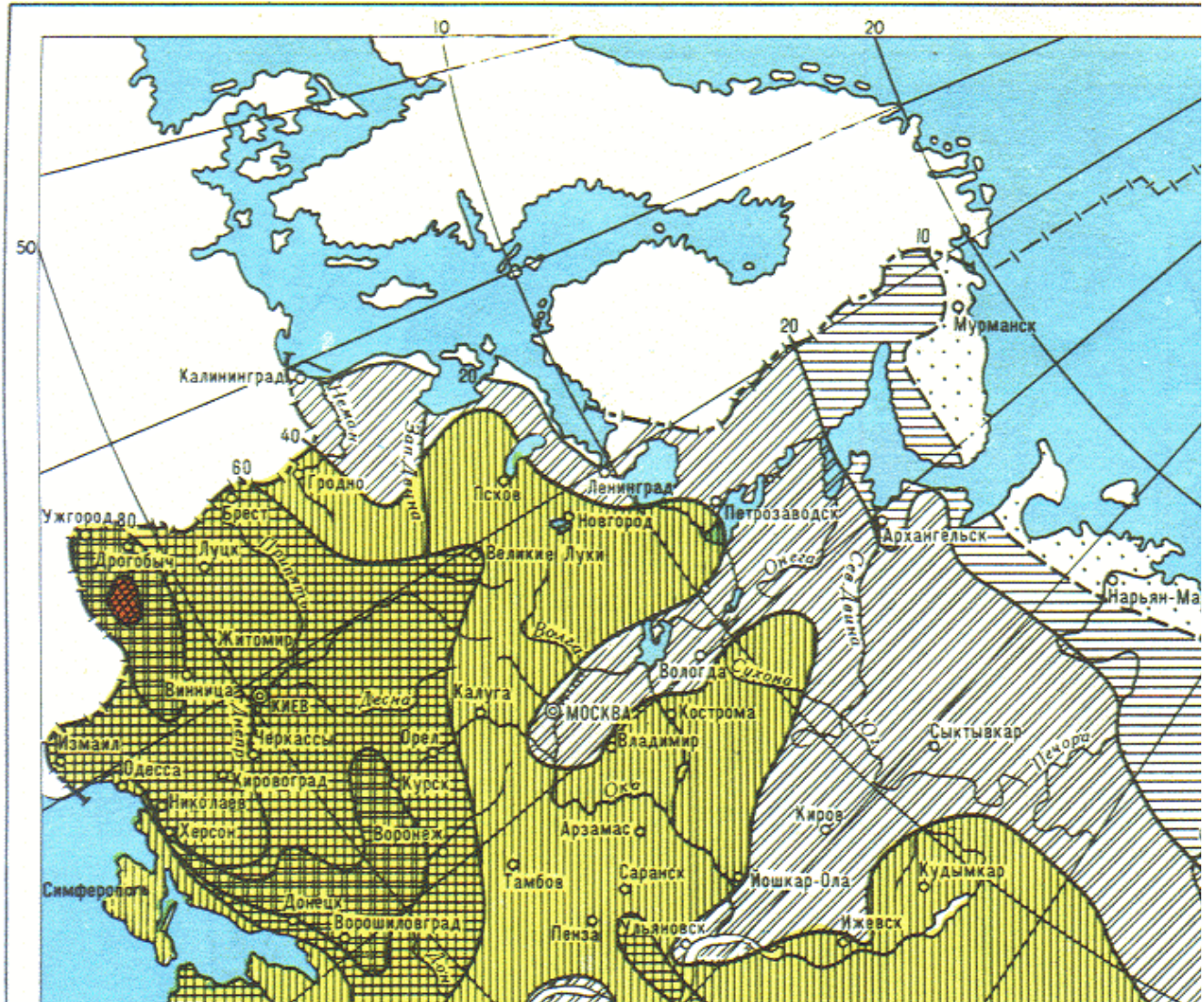
Рис. 2.5.13. Карта среднегодовой продолжительности гроз. Лист 1
